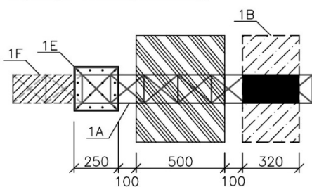
Půdorys jeřábu (Obr. 2)
